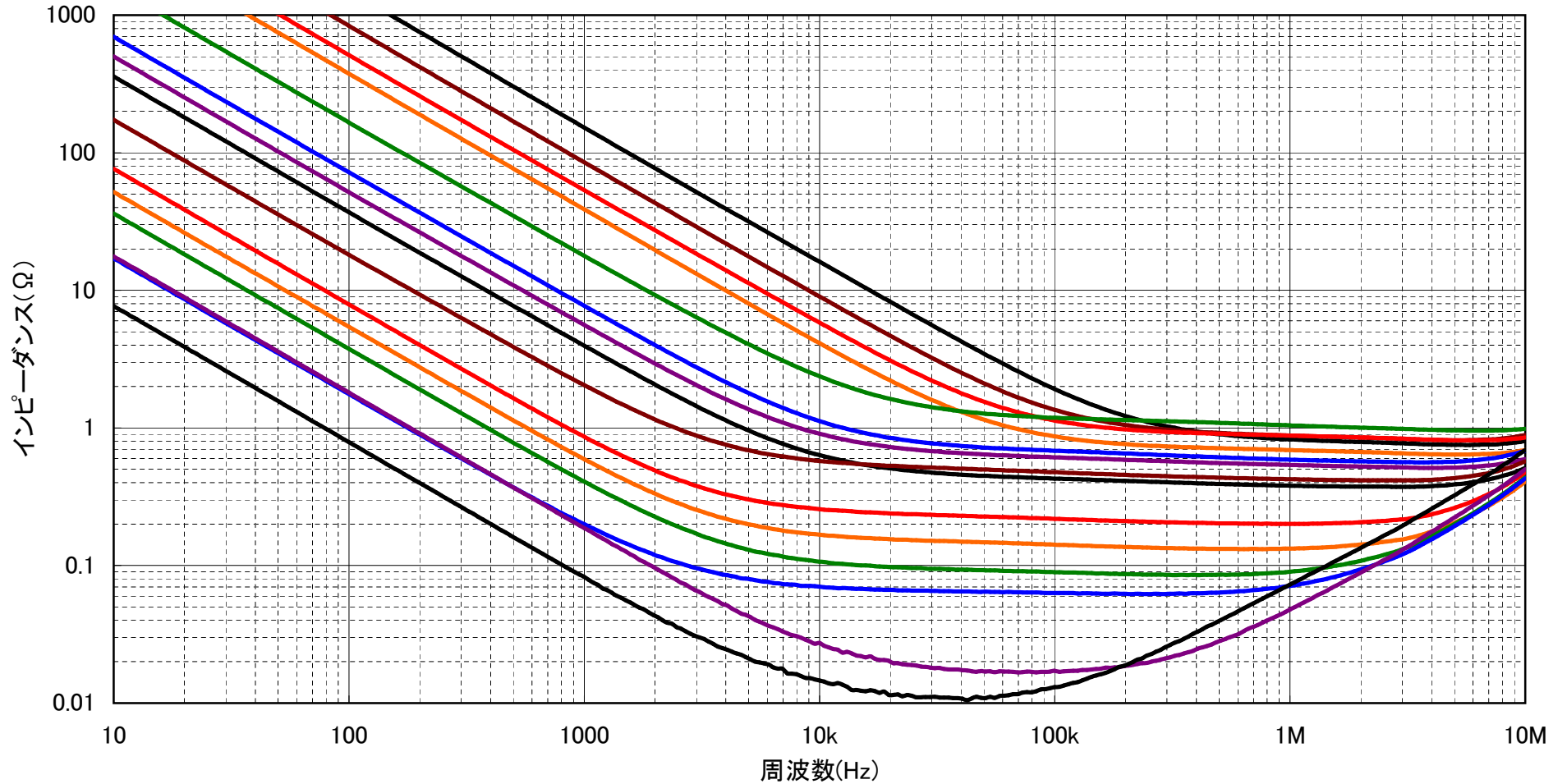
Rubycon 電解コンデンサ YK インピーダンス-周波数特性
