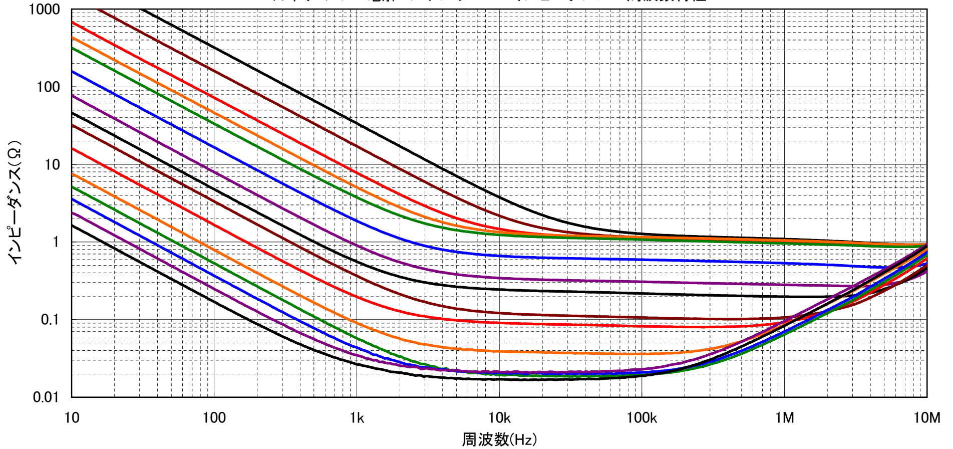
日本ケミコン 電解コンデンサ SMG インピーダンス-周波数特性
