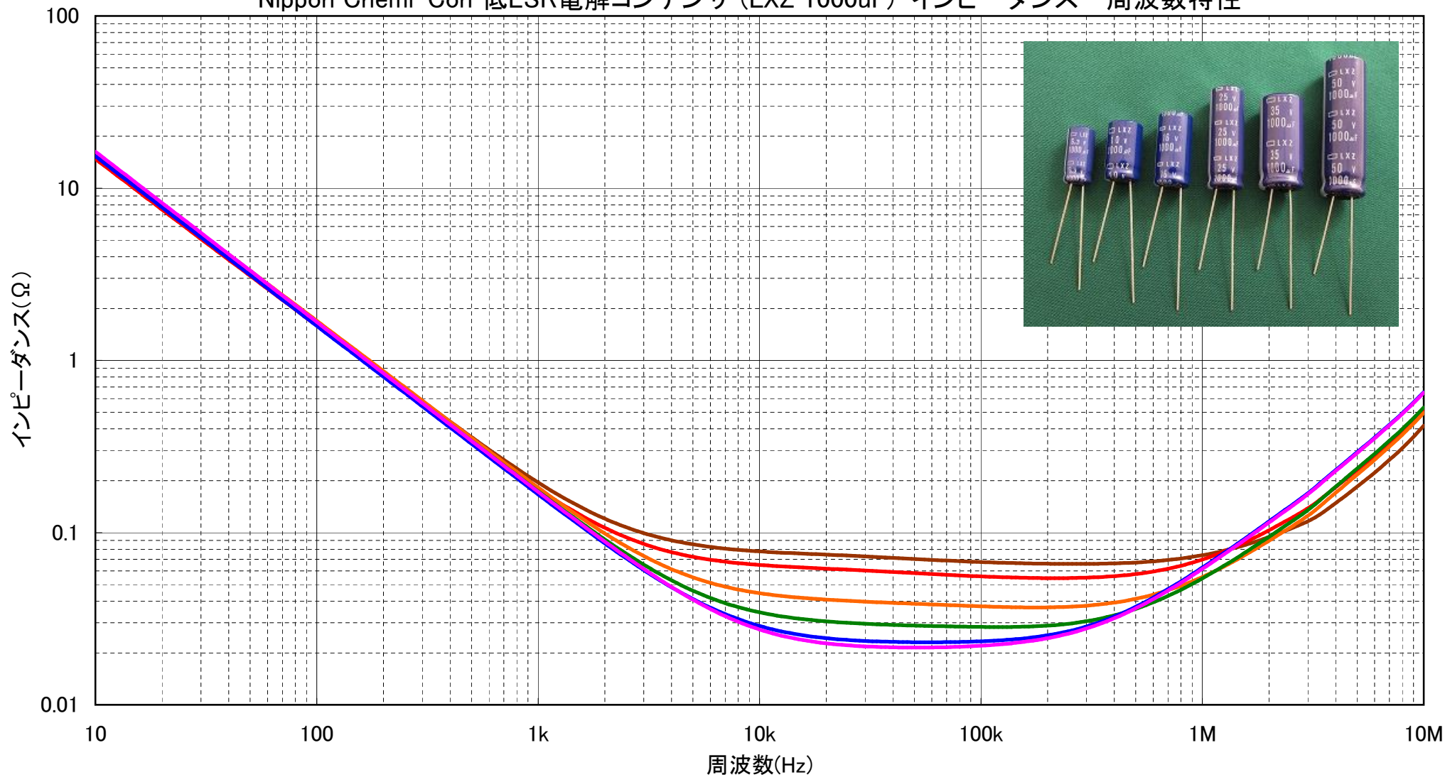
Nippon Chemi-Con 低ESR電解コンデンサ (LXZ 1000uF) インピーダンスー周波数特性
