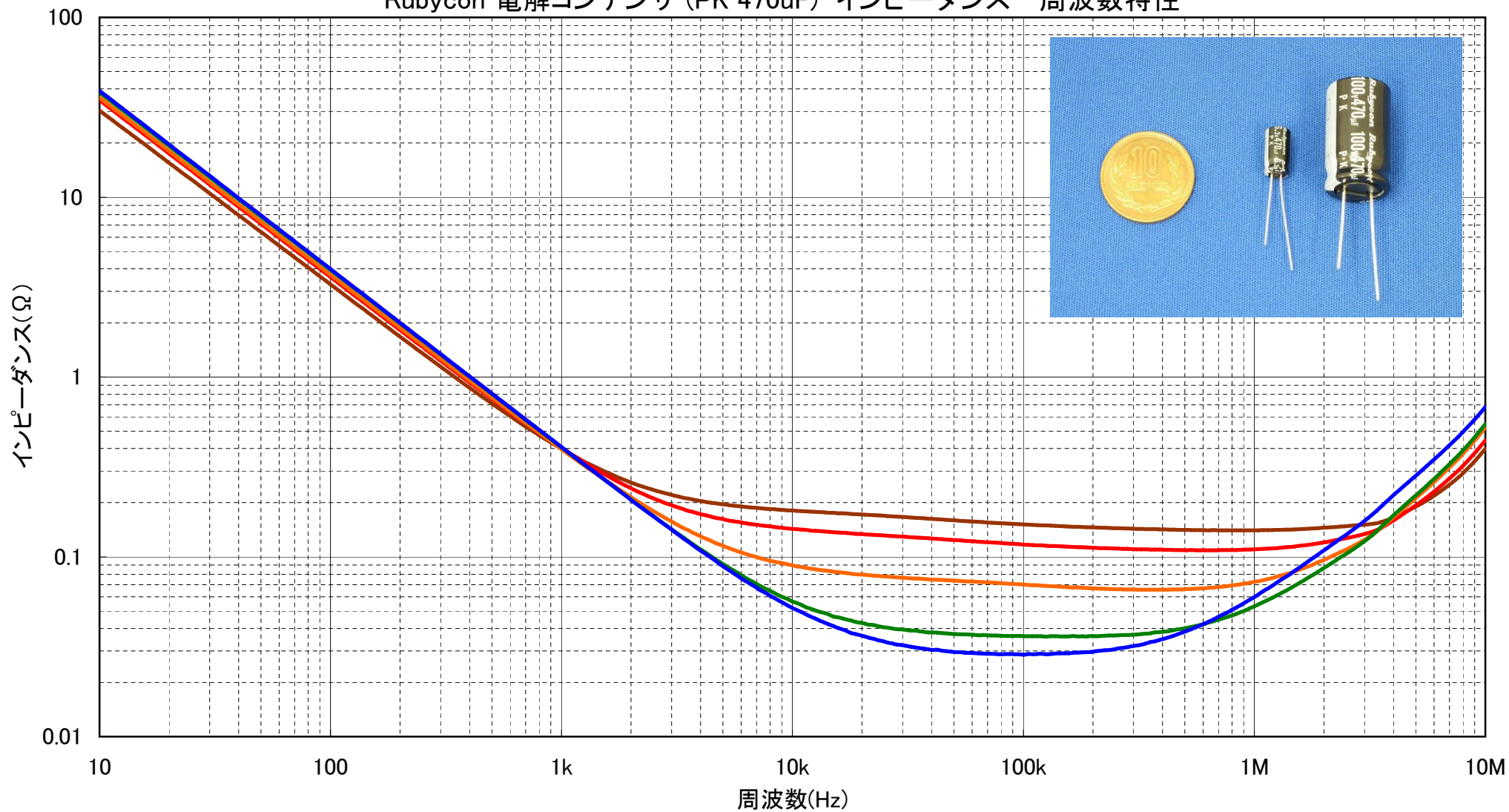
Rubycon 電解コンデンサ (PK 470uF) インピーダンス-周波数特性
