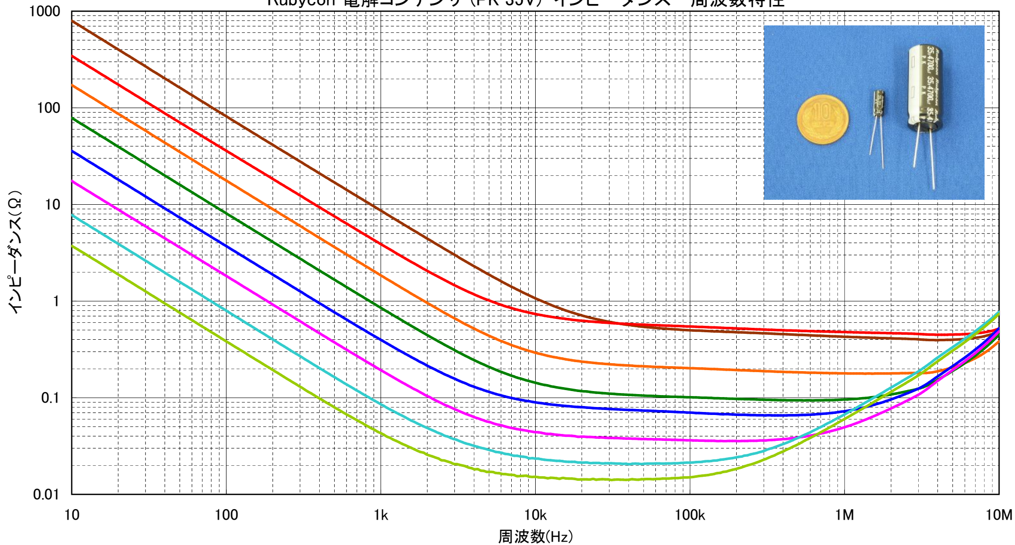
Rubycon 電解コンデンサ (PK 35V) インピーダンス-周波数特性
