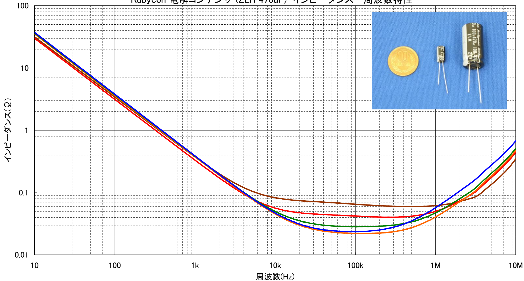
Rubycon 電解コンデンサ (ZLH 470uF) インピーダンス-周波数特性
