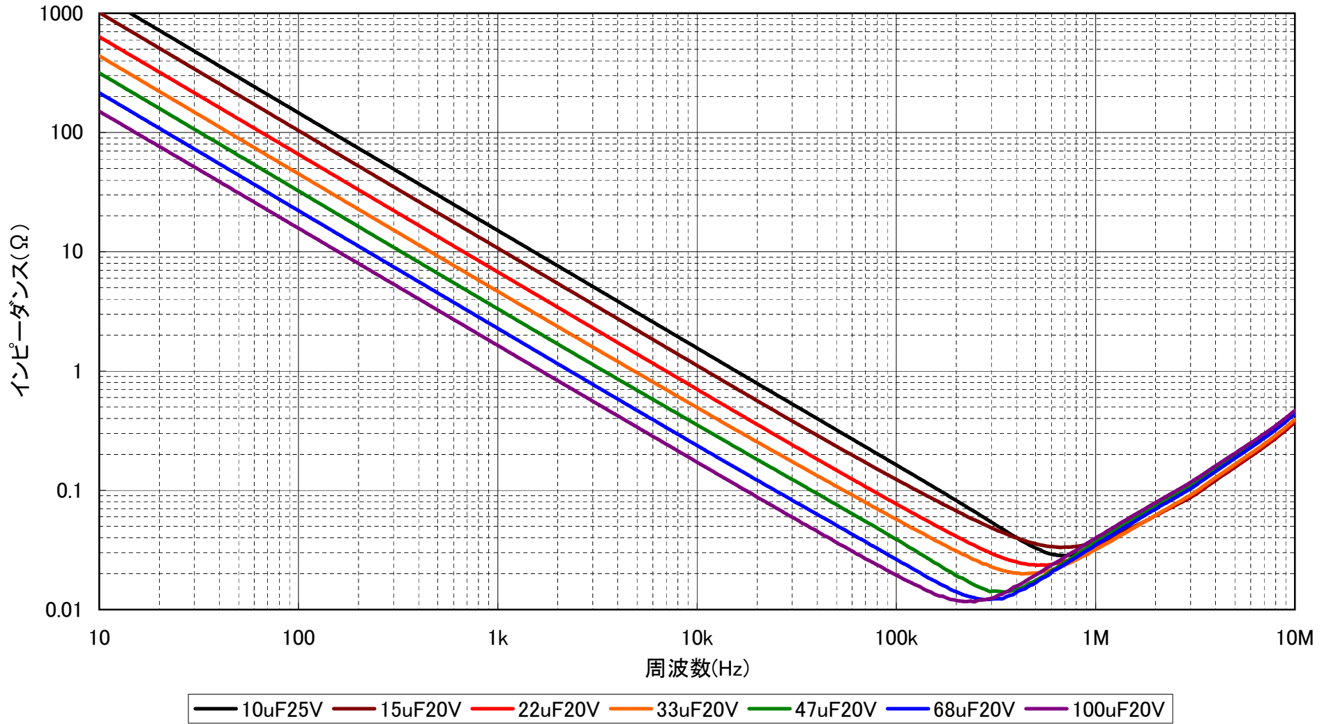
有機半導体アルミ固体電解コンデンサSH20V,25Vのインピーダンス周波数特性
