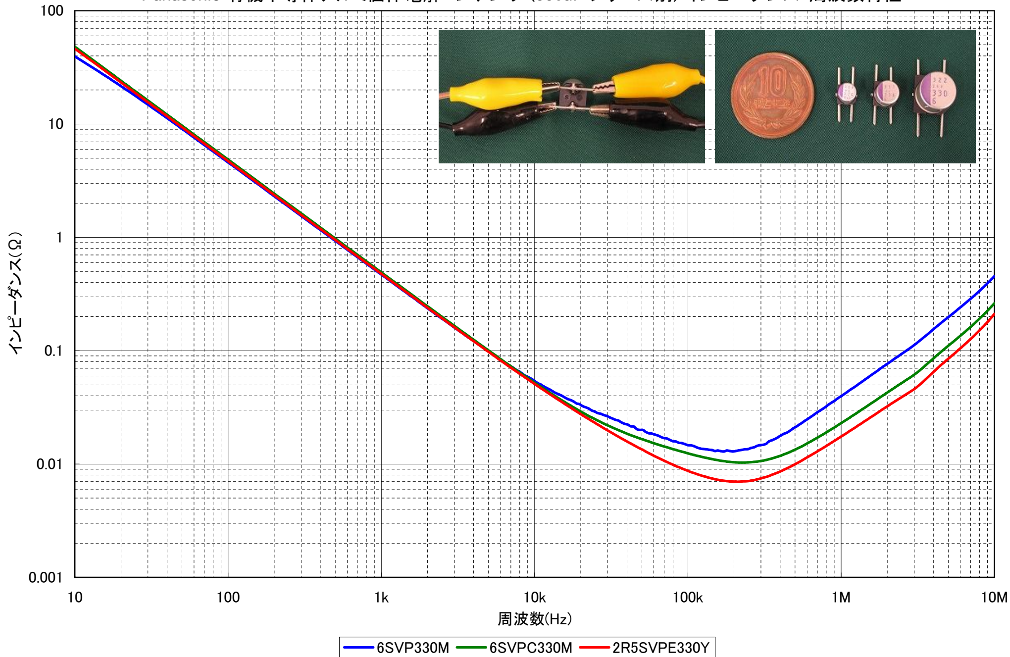
Panasonic 有機半導体アルミ個体電解コンデンサ (330uF シリーズ別) インピーダンス-周波数特性
