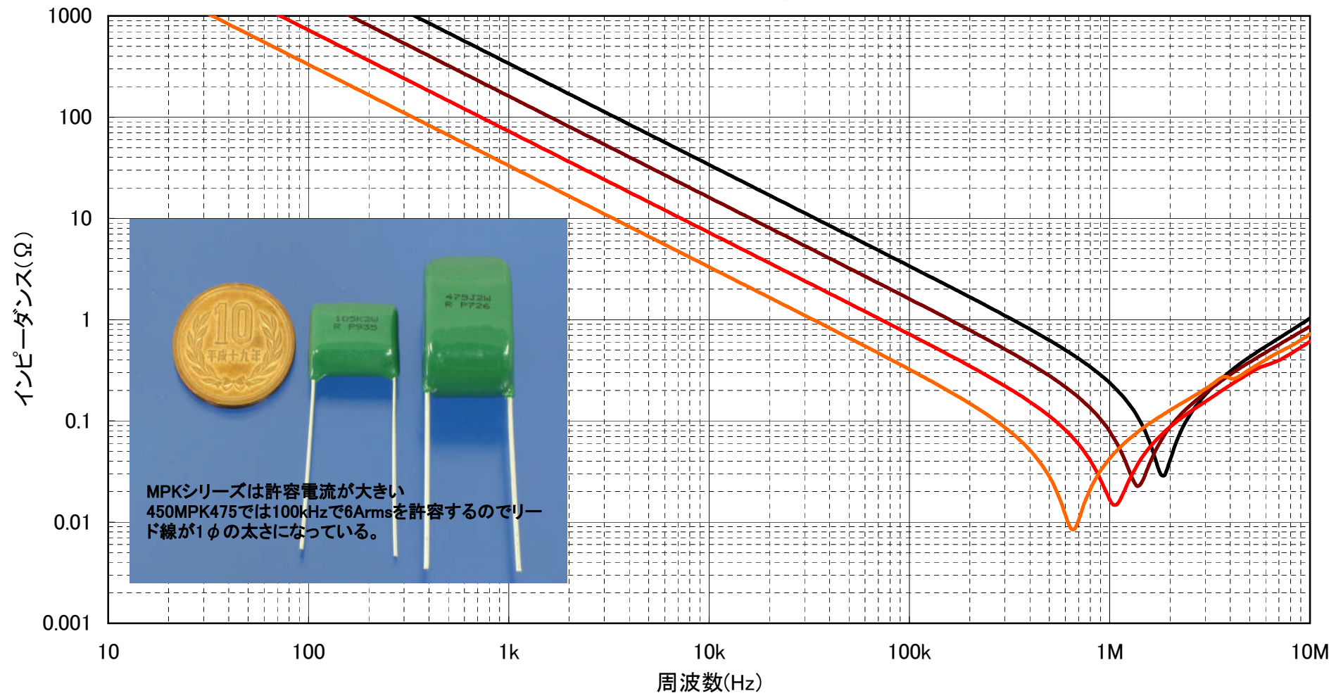
メタライズド・ポリプロピレン・フィルム・コンデンサ(Rubycon MPK)のインピーダンス周波数特性
