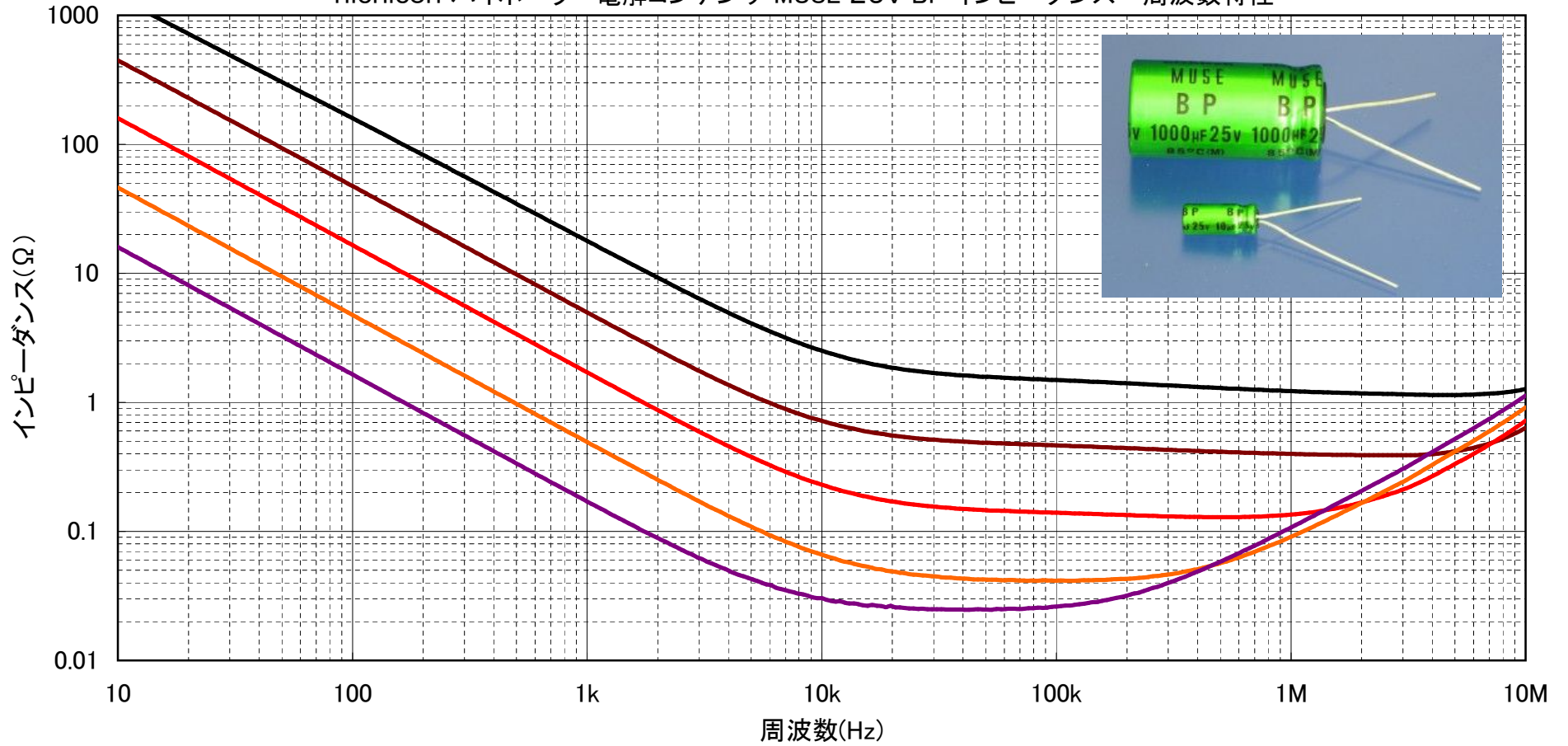
nichicon バイポーラー電解コンデンサ MUSE 25V BP インピーダンス-周波数特性
