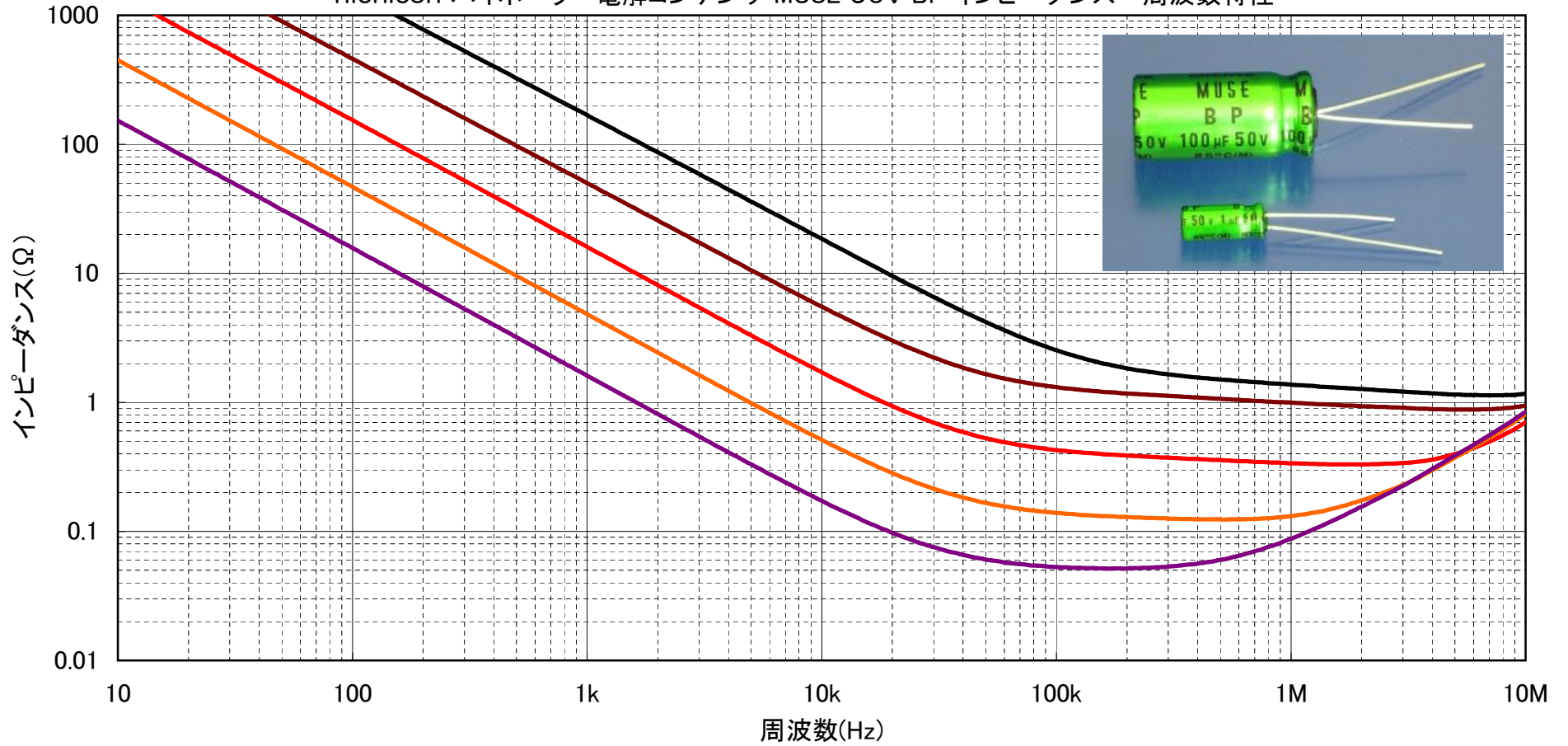
nichicon バイポーラー電解コンデンサ MUSE 50V BP インピーダンス-周波数特性
