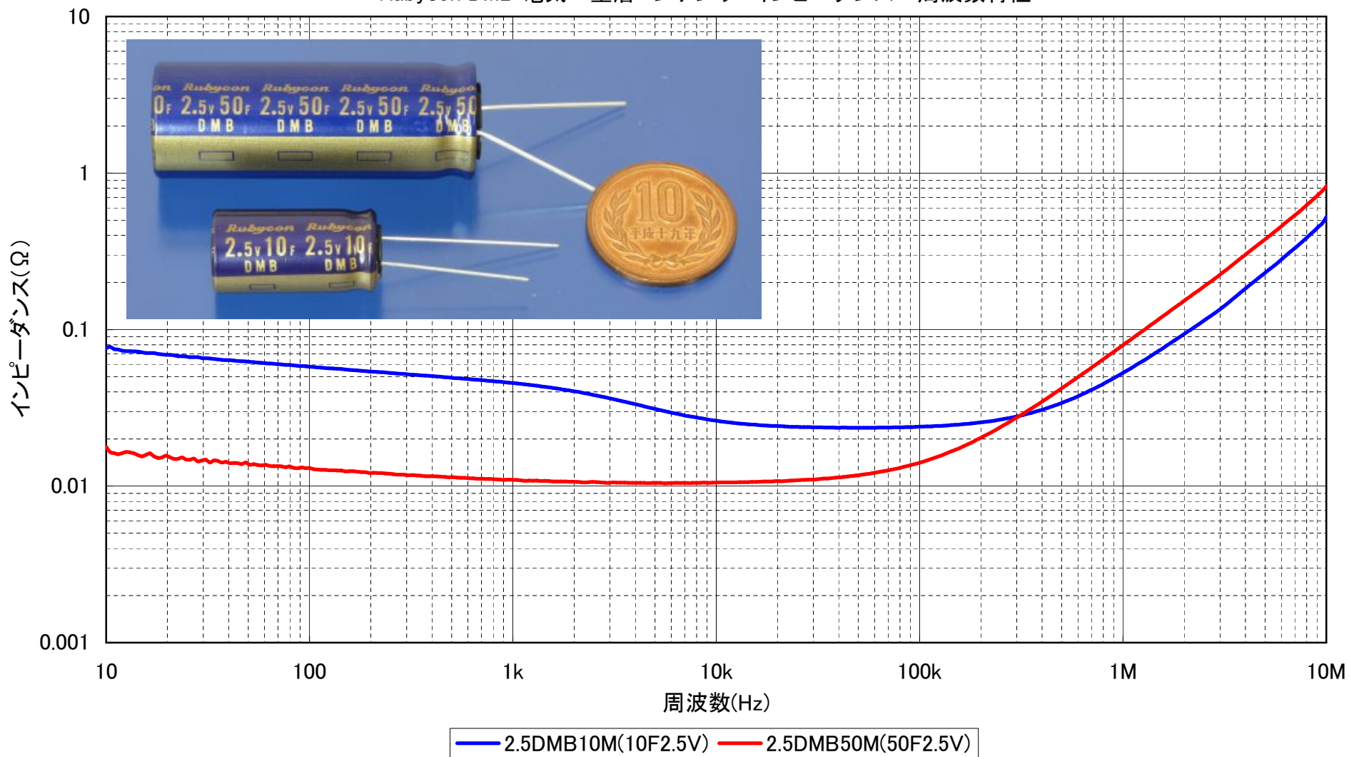
Rubycon DMB 電気二重層コンデンサ インピーダンスー周波数特性
