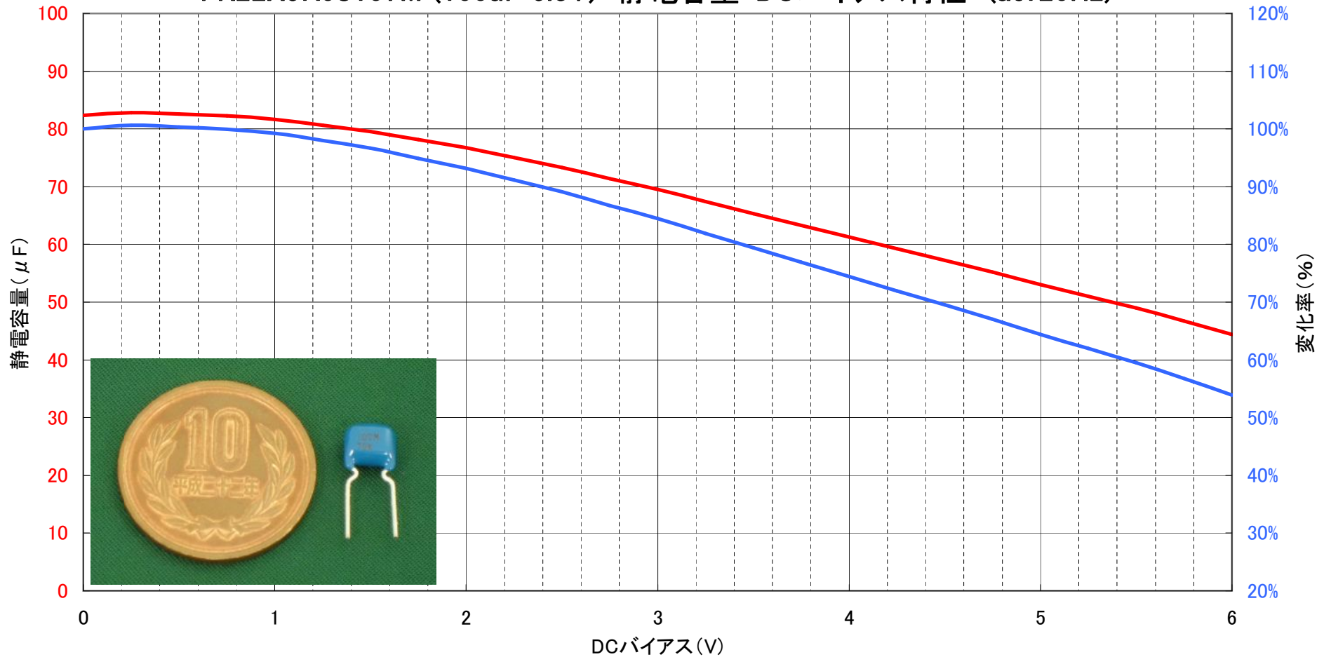
FK22X5R0J107M (100 \mu F 6.3V) 静電容量-DCバイアス特性 (at120Hz)
