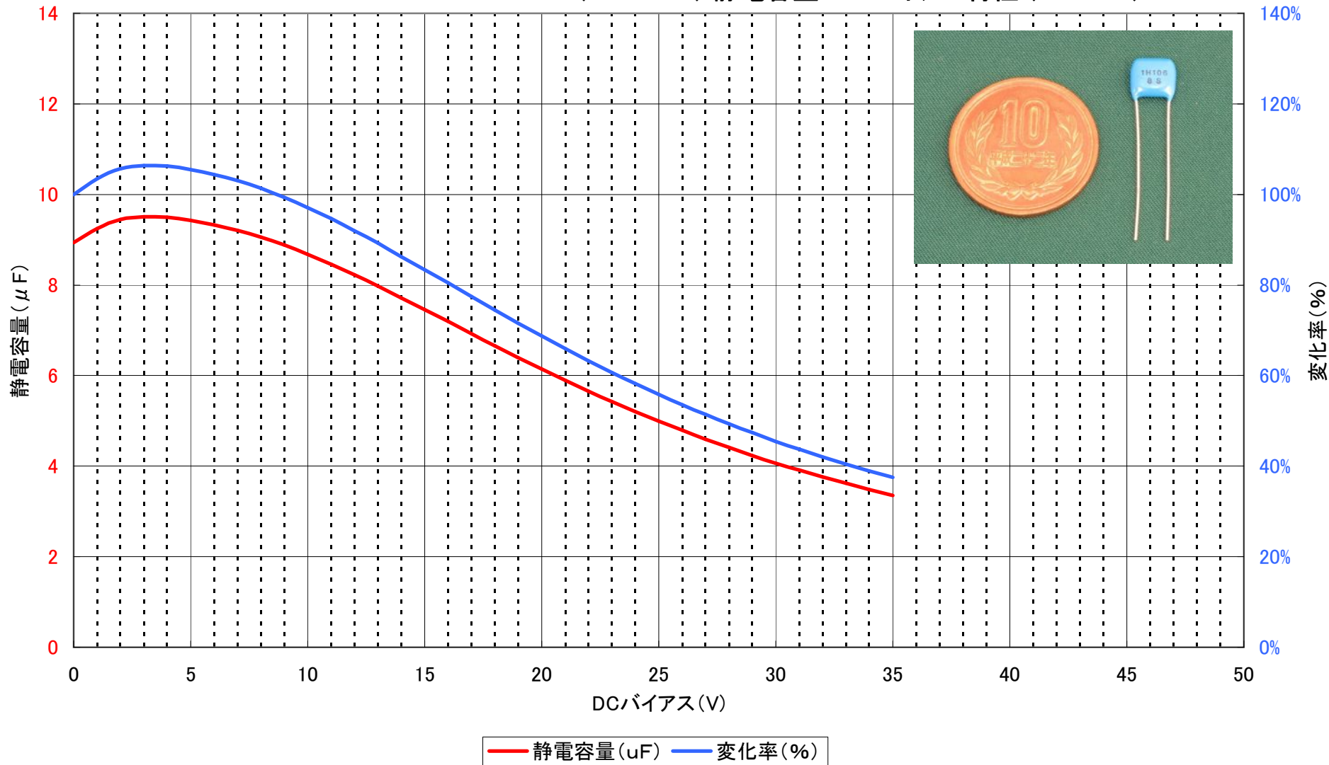
NIPPON CHEMI-CON THD31H106Z (10 \mu F 50V) 静電容量-DCバイアス特性 (at10KHz)
