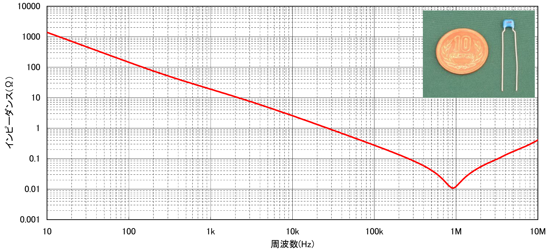
Supertech RD20F106Z1EH5L(Y5V) 積層セラミックコンデンサ インピーダンス—周波数特性
