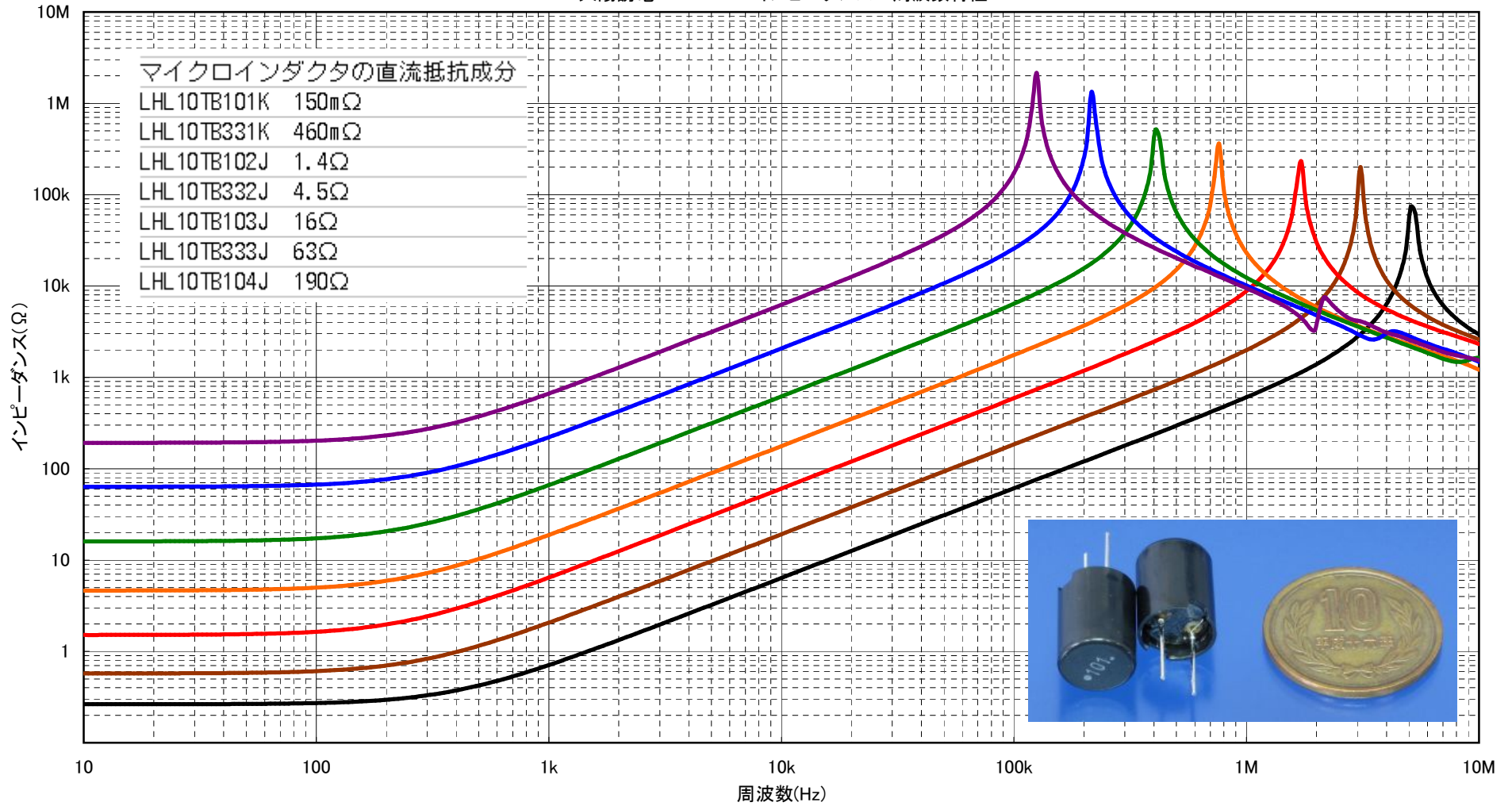
大陽誘電 LHL10TB インピーダンス-周波数特性
