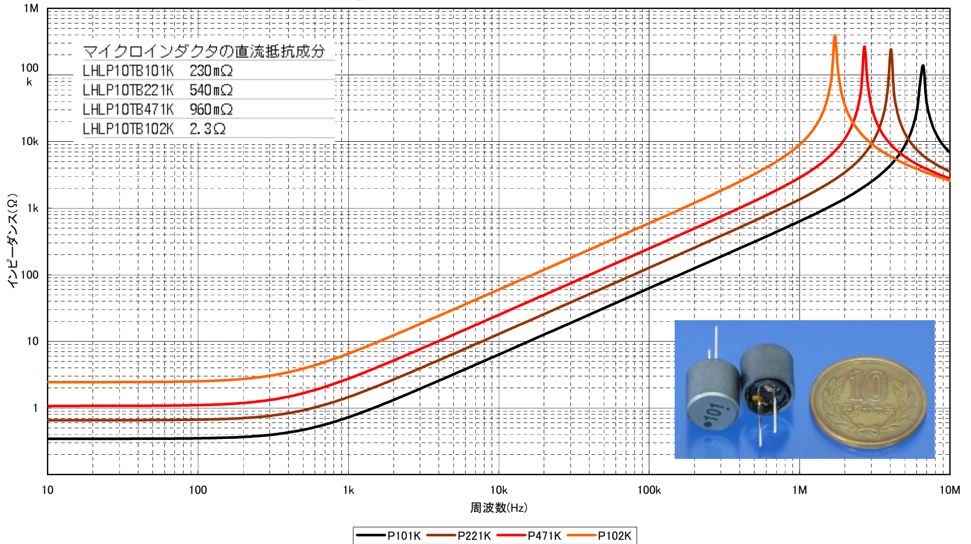
大陽誘電 LHL10TB(磁気シールドタイプ) インピーダンス-周波数特性
