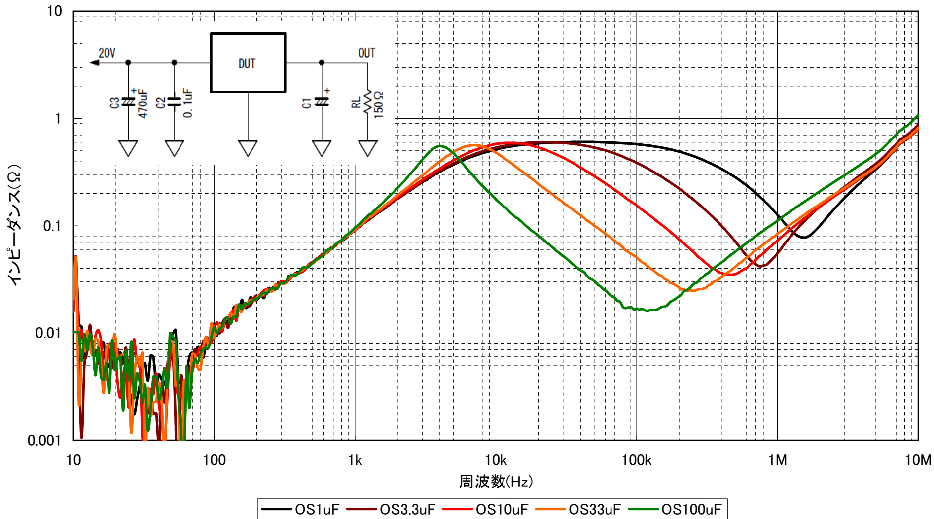
NJM7815FA 出力コンデンサ(OSコンデンサ)による出カインピーダンスの変化
