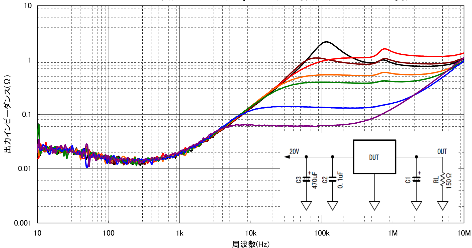
LDO LM2940-15 出力コンデンサ(Rubycon YK)による出カインピーダンスの変化
