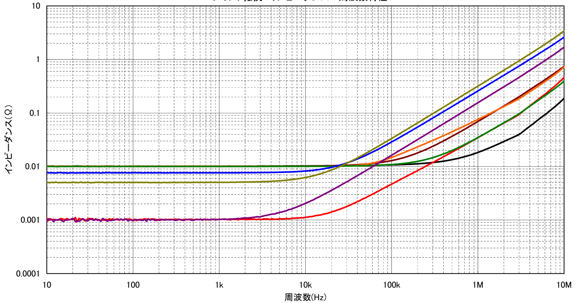
シャント抵抗 インピーダンス-周波数特性
