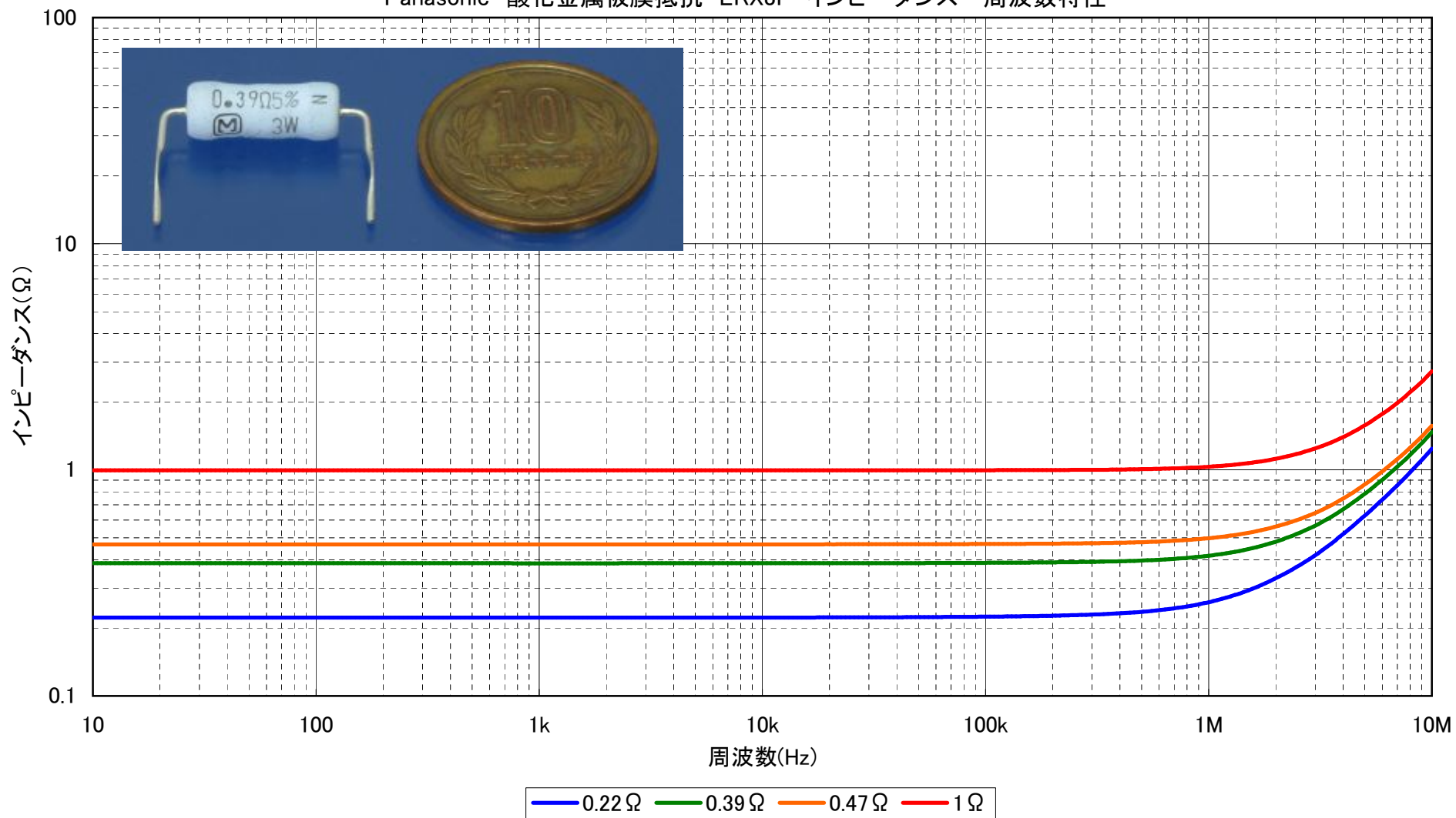
Panasonic 酸化金属被膜抵抗 ERX3F インピーダンス-周波数特性
